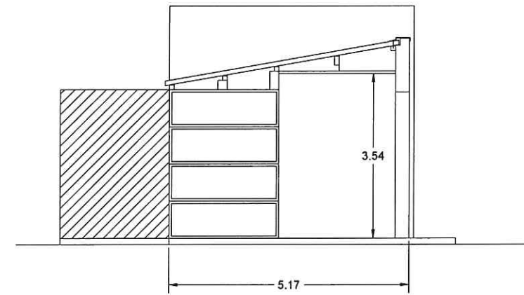
SEZIONE A-A
